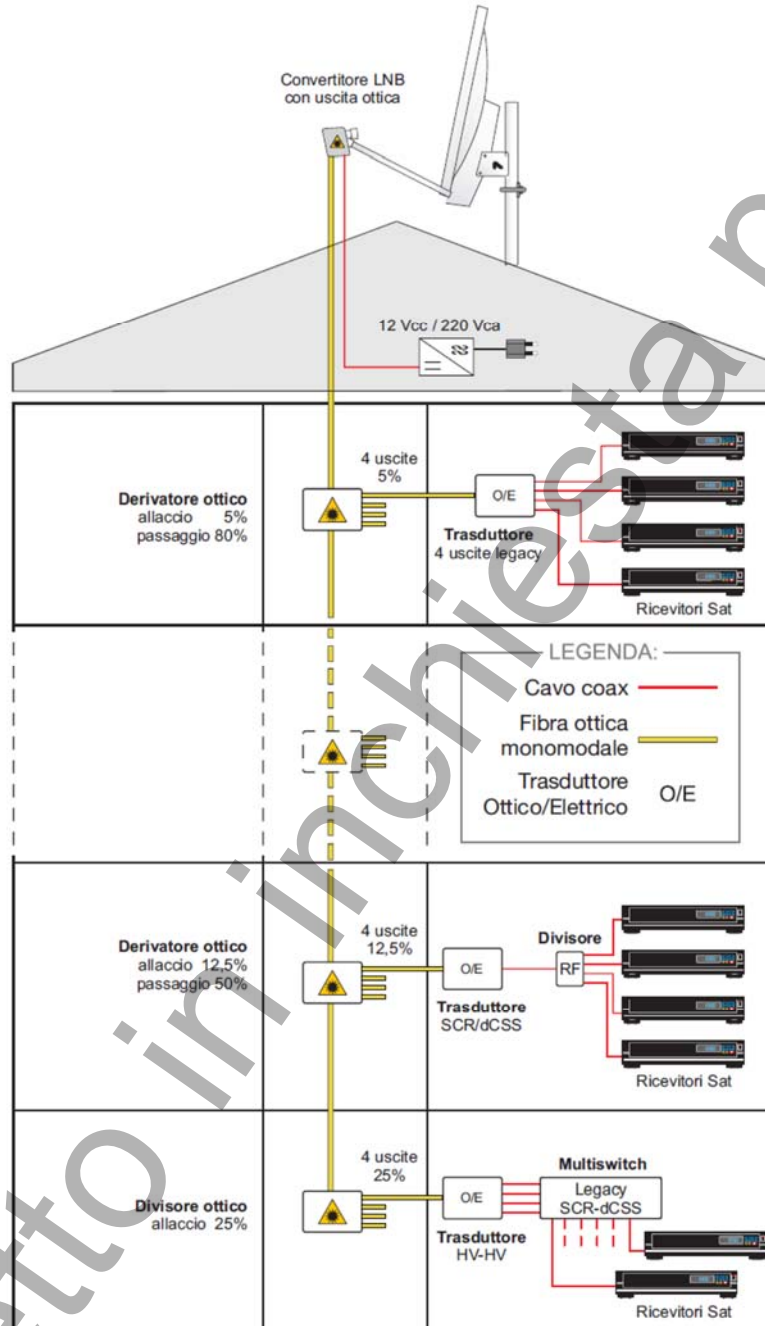
Figura 19 – Esempio di distribuzione segnali TV SAT con montante ottico e distribuzione interna su cavo coassiale
