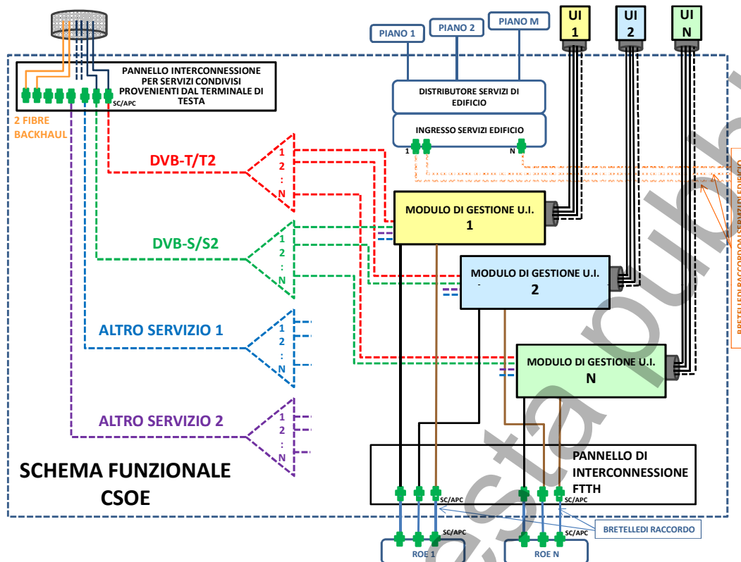
Figura 41 – Esempio di CSOE per un edificio a M piani e N unità immobiliari predisposto per implementazioni future
