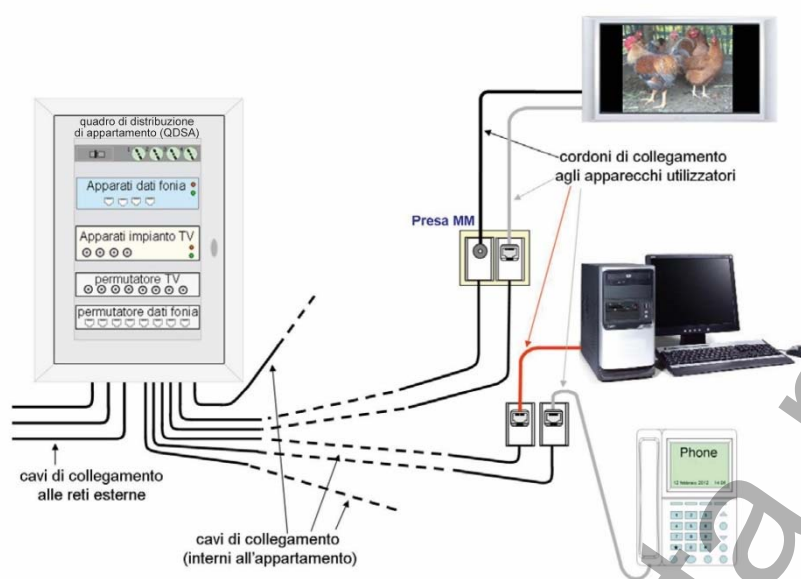
Figura 11 – Schema di collegamento tra quadro di distribuzione e punti di utilizzo
