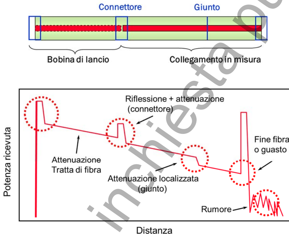
Figura 72 – Esempio di misura riflettometrica e relativa traccia
