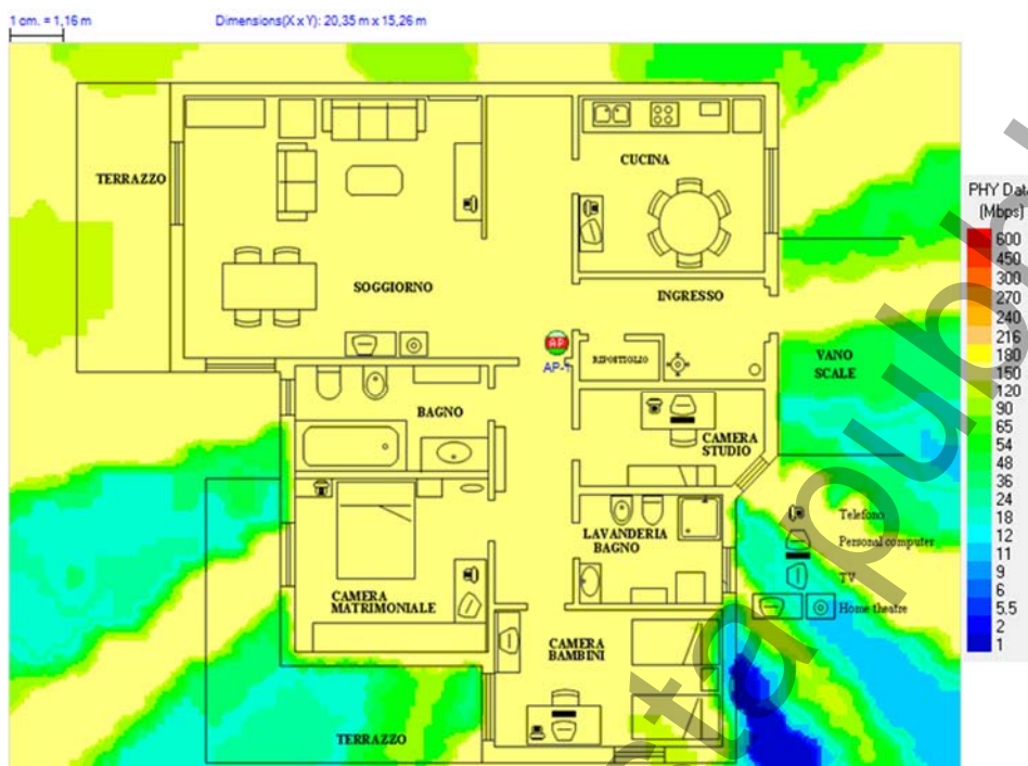
Figura 15 – Prestazioni a livello fisico dell'AP con bit rate massimo 150 Mb/s
