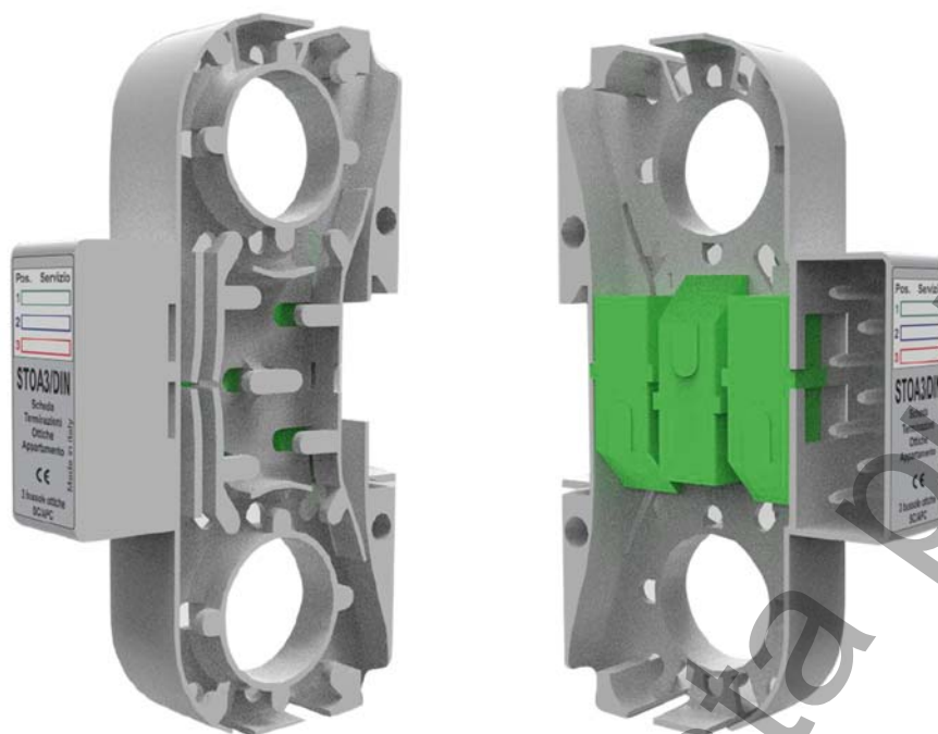
Figura 45 – Esempio di STOA per barra DIN con 3 bussole scalabili (6,9...)
