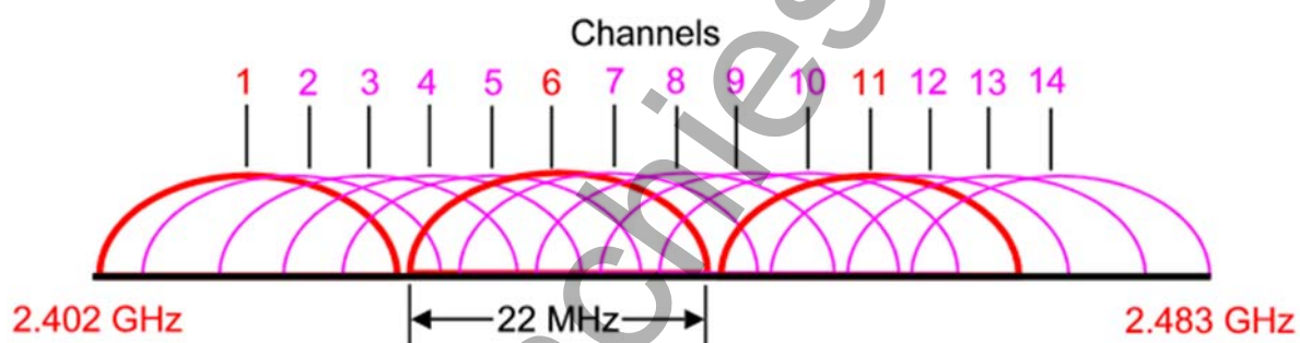
Figura 13 – Dettaglio sulla caratterizzazione della banda Wi-Fi 2,4 GHz
