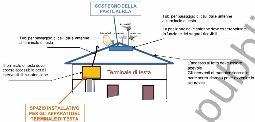
Figura 32 – Rappresentazione schematica del punto di accesso all'edificio per segnali via radio nel caso di installazioni condominiali
