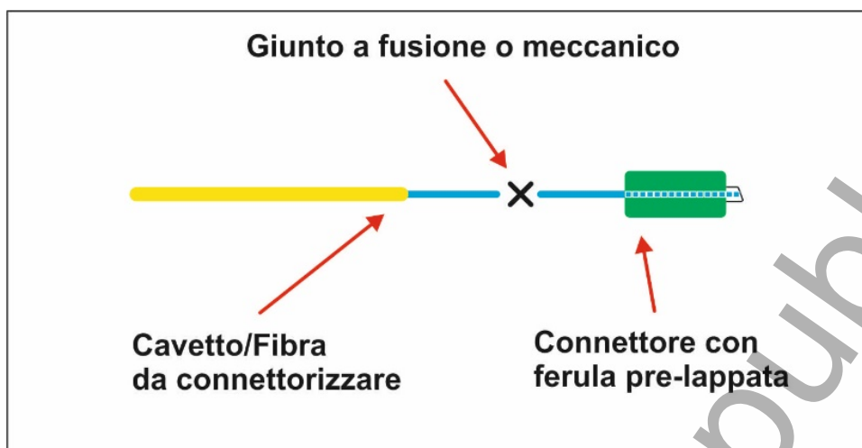
Figura 55 – Connettorizzazione in campo
