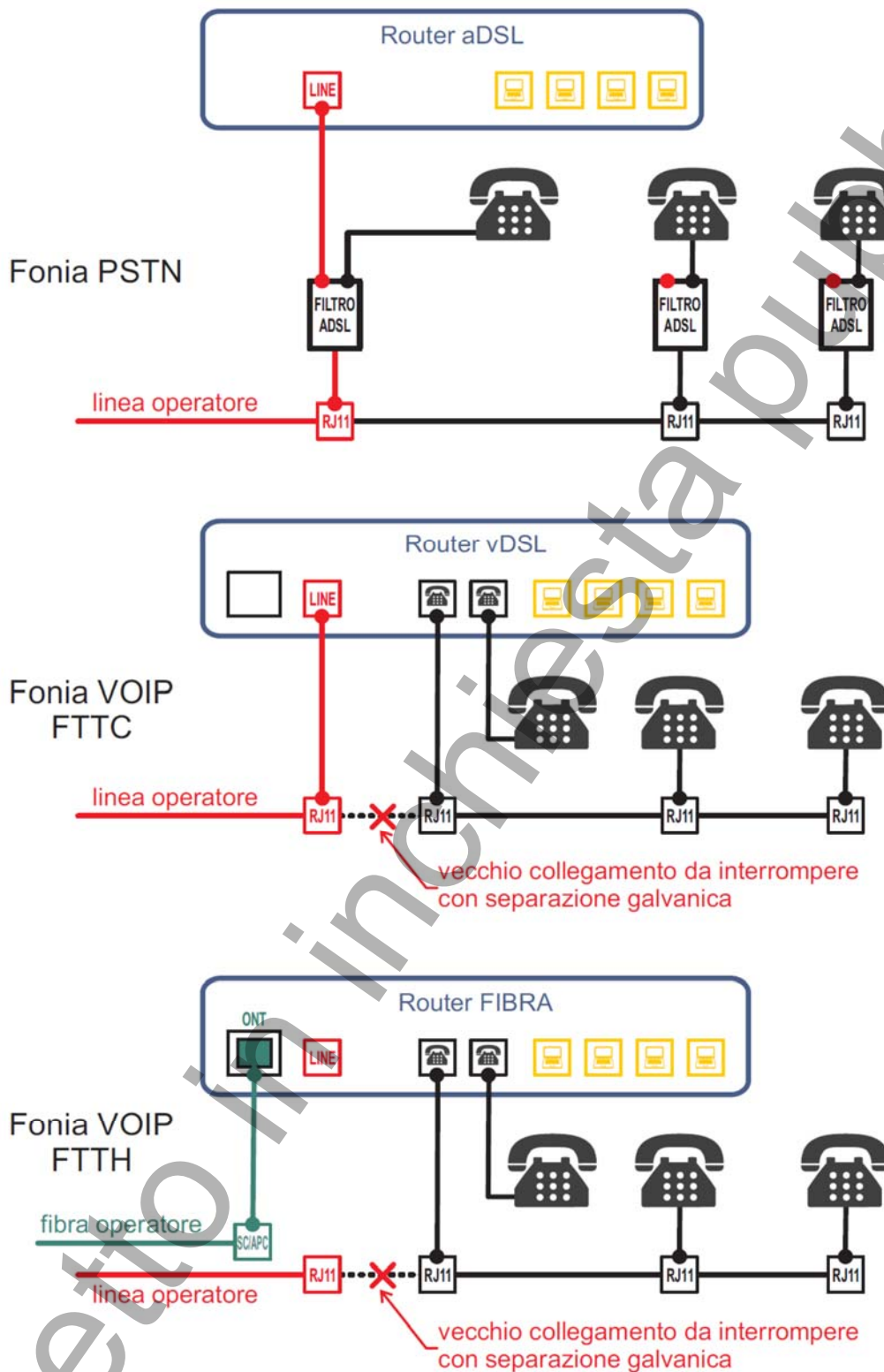
Figura 4 – Schemi di collegamento rete di distribuzione della fonia nei casi di ADSL, VDSL, FTTH
