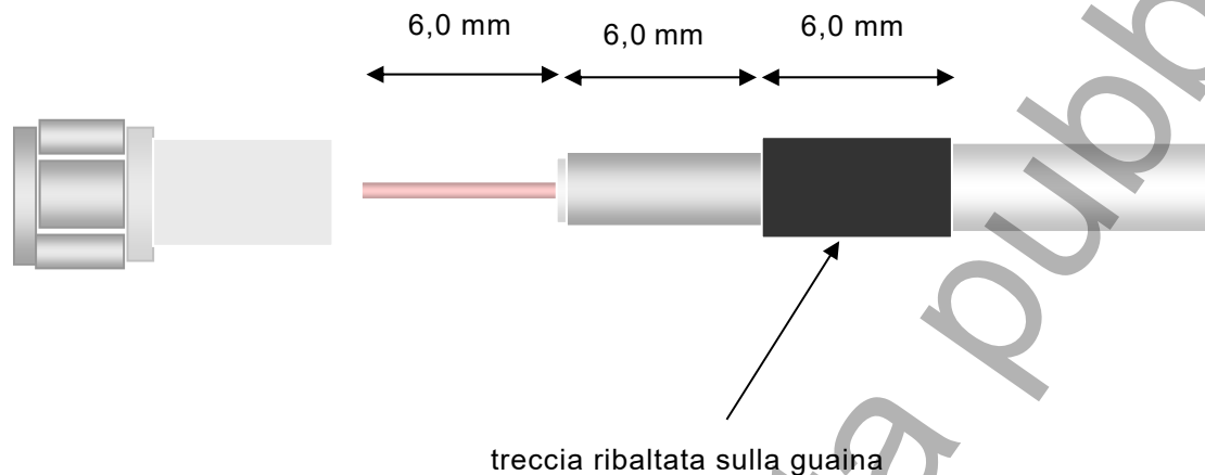
Figura 66 – Installazione di un connettore F fase 2
