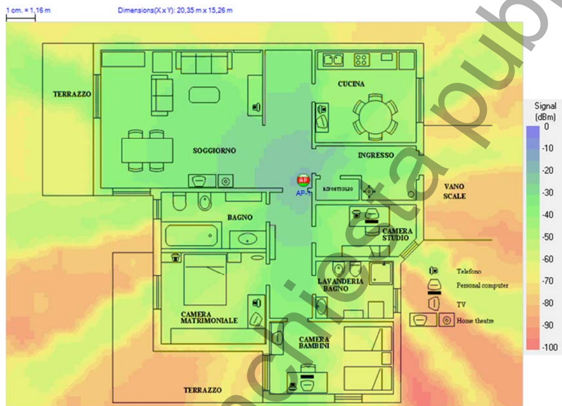
Figura 14 – Simulazione area di copertura di un AP IEEE802.11 con canale a 20 MHz e con max MCS15
