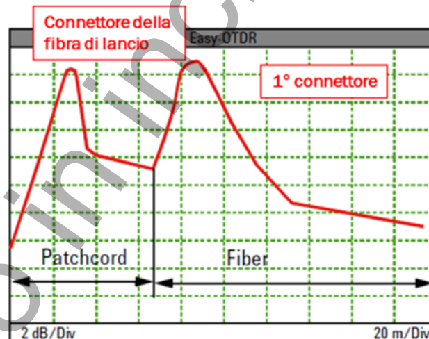
Figura 73 – Traccia OTDR- Esempio 1
