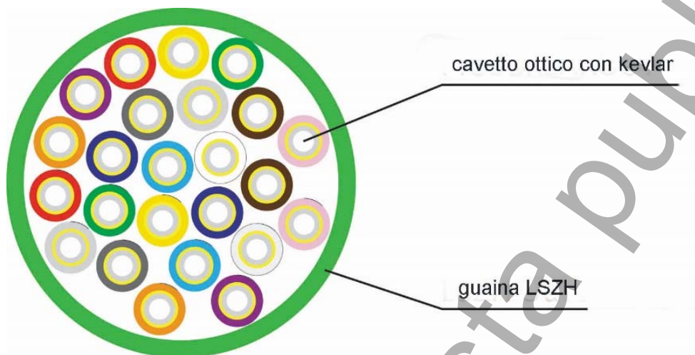
Figura 48 – Esempio di cavo multifibra a struttura lasca
