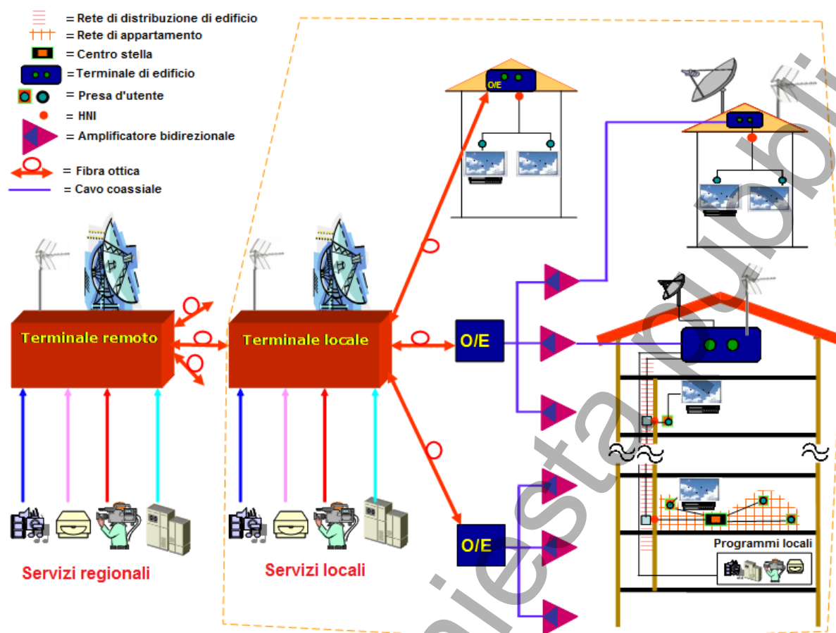
Figura 51 Struttura dell' impianto TV per un comprensorio
