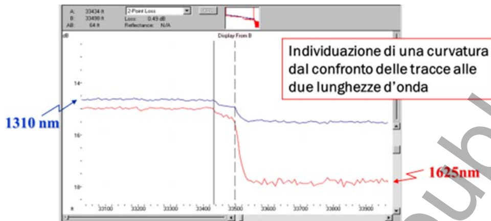
Figura 77 – Traccia OTDR - Esempio 5
