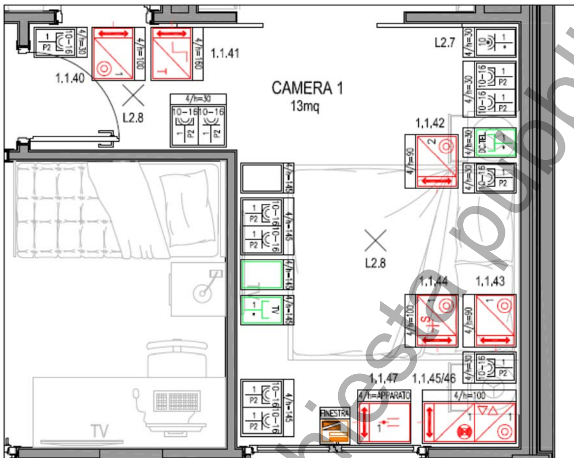
Figura 85 – Dettaglio camera da letto matrimoniale
