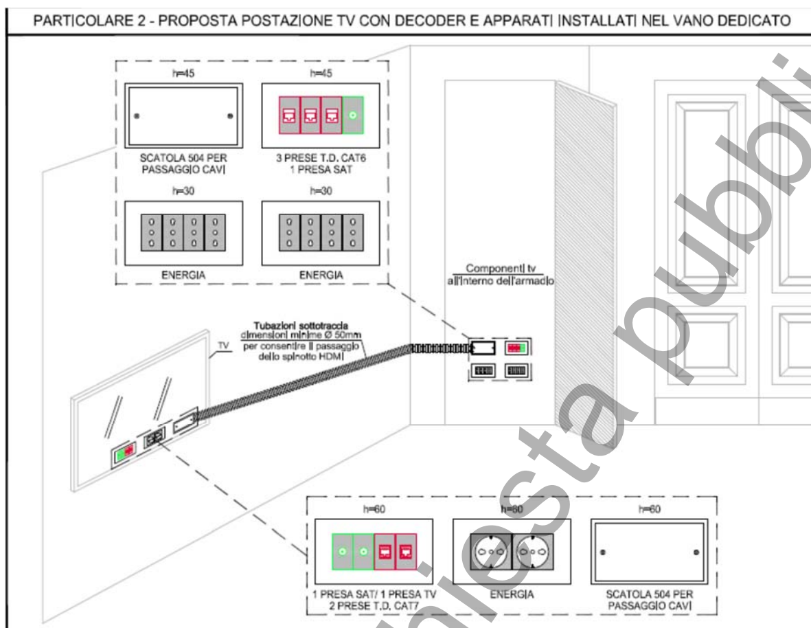
Figura 88 – Dettaglio postazione TV con spazio dedicato per decoder e apparati
