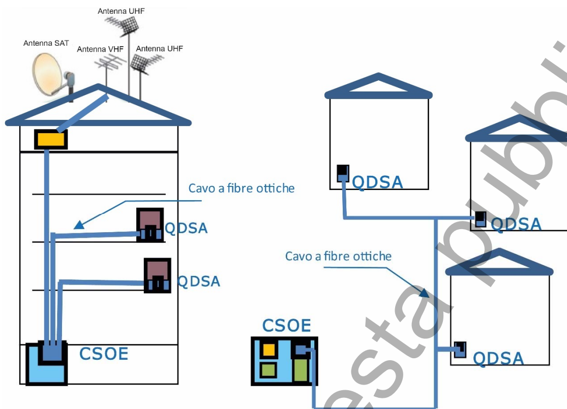
Figura 40 – Rappresentazione schematica dell'impianto di comunicazione in fibra ottica nel caso di edifici a distribuzione verticale e orizzontale
