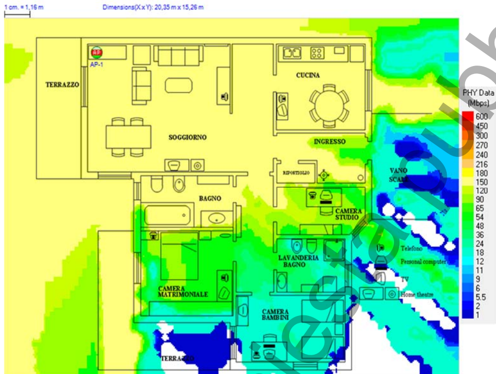
Figura 17 – Prestazioni di un AP con diagramma di irradiazione isotropo collocato in maniera non ottimale
