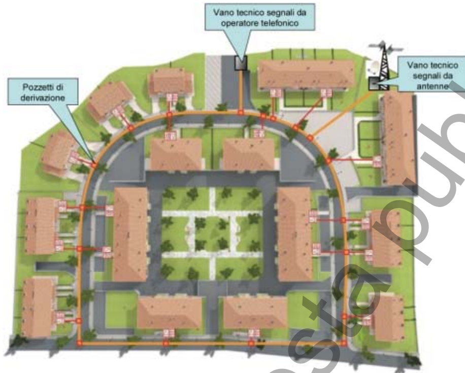
Figura 25 – Esempio di predisposizione infrastrutturale in caso di unità immobiliari distribuite orizzontalmente
