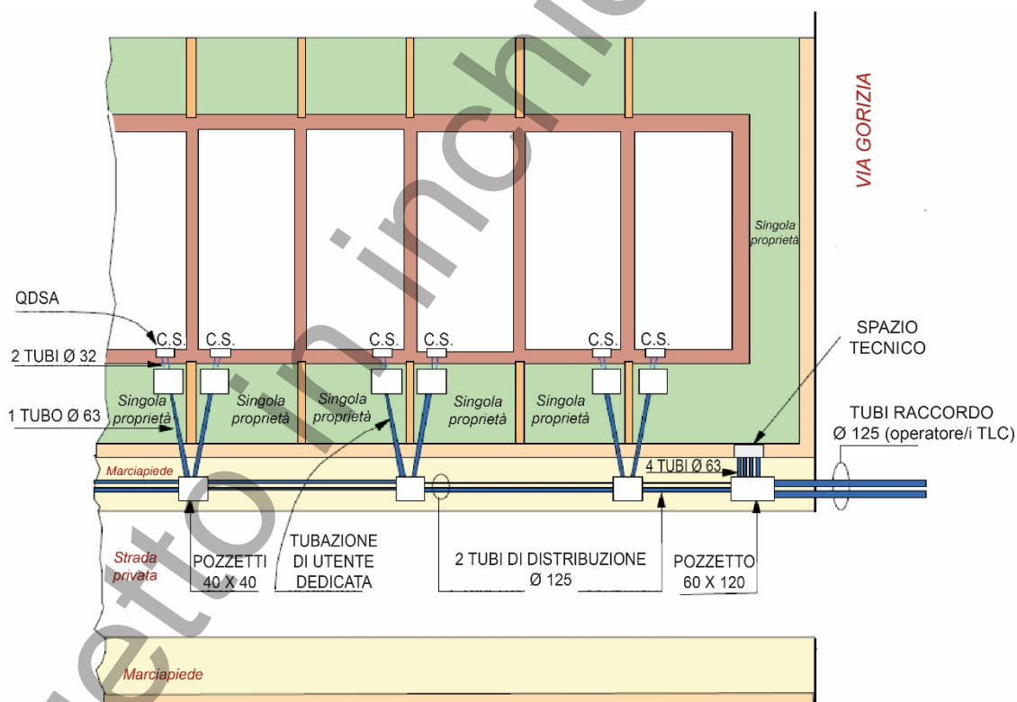
Figura 24 – Esempio di infrastrutture in caso di unità immobiliari distribuite appartenenti ad un complesso immobiliare unico
