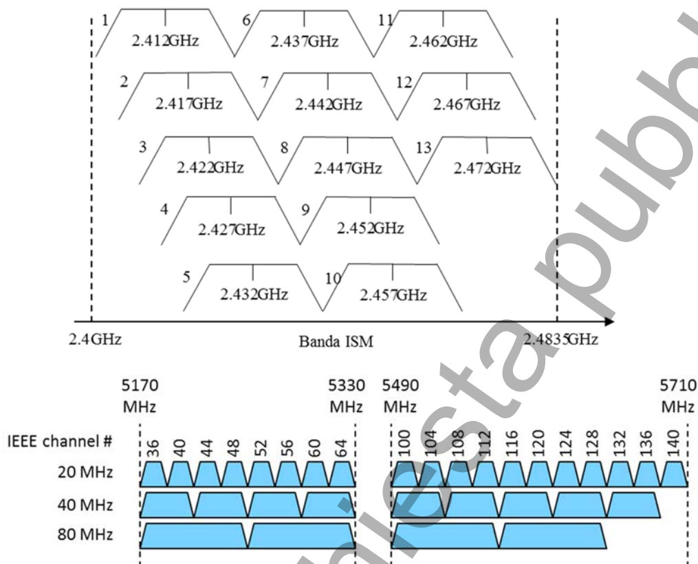
Figura 12 – Canali Wi-Fi e rispettive frequenze nelle bande 2,4 GHz e 5 GHz
