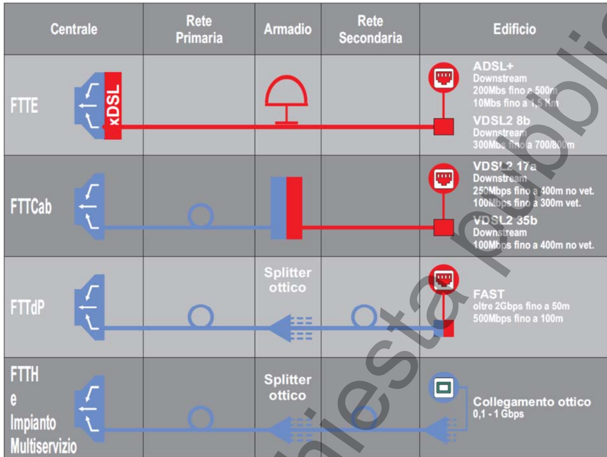
Figura 5 – Architettura di rete di accesso fisso
