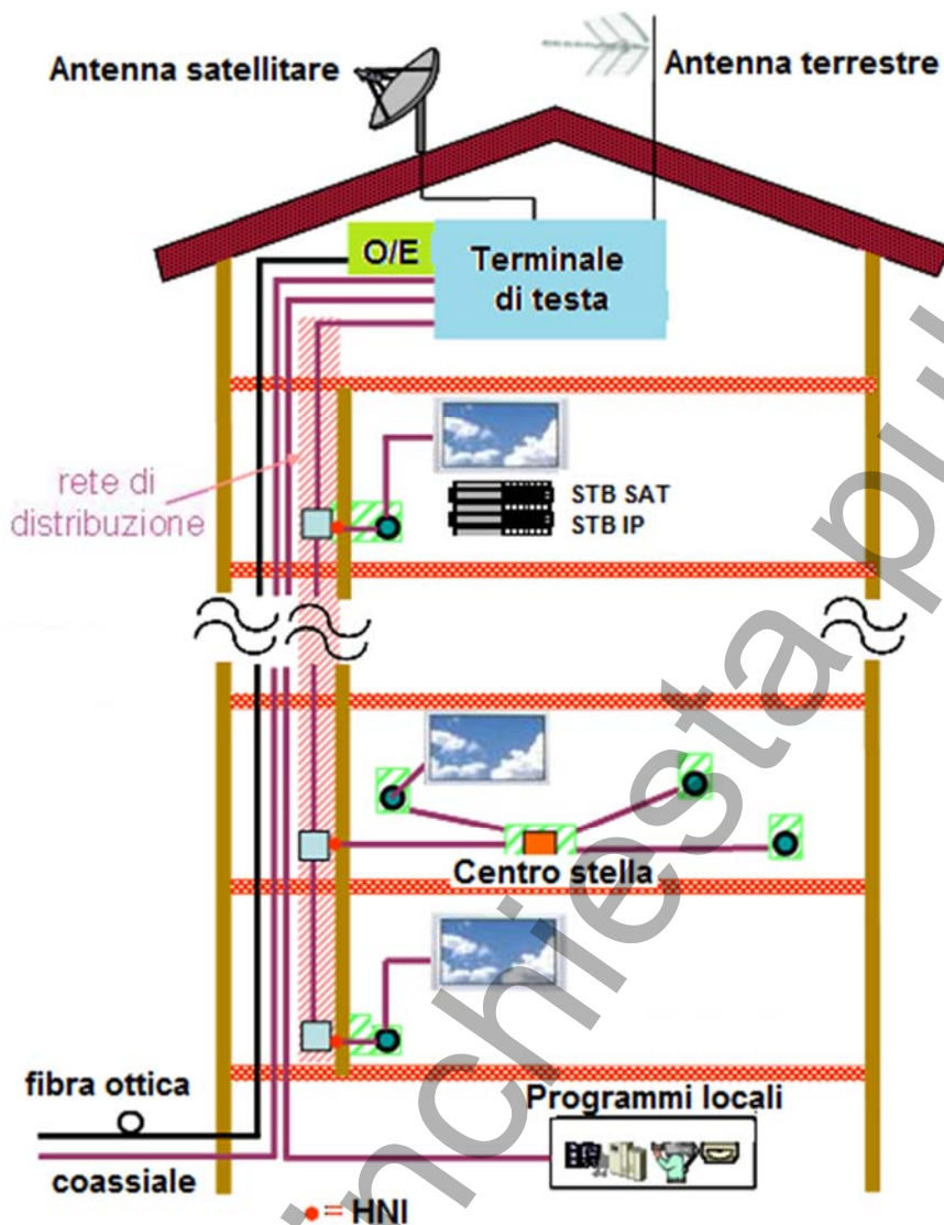
Figura 50 – Struttura dell'impianto TV in un edificio
