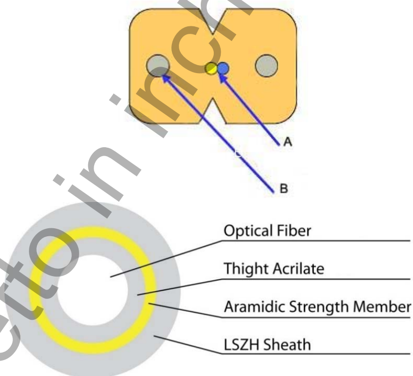
Figura 49 – Esempio di cavi compatti per il collegamento verticale e/o orizzontale di edificio (sez. rettangolare: bi-fibra; circolare: mono-fibra)
