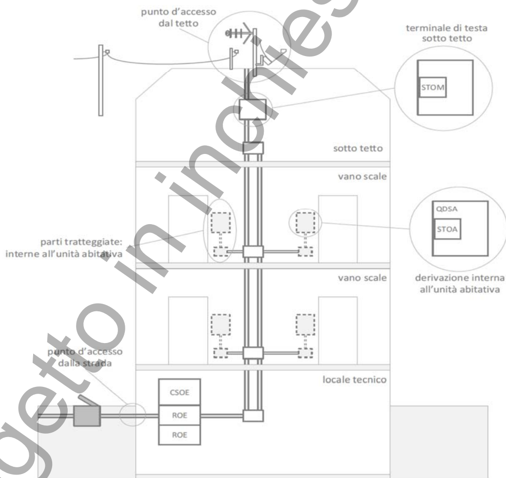
Figura 26 – Rappresentazione schematica delle zone di accesso all'edificio nel caso di reti provenienti sia dalla strada sia del tetto (CSOE alla base si veda cap. 8)
