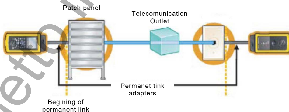
Figura 67 – Verifica dei parametri di trasmissione (Fonte: Fluke Networks)
