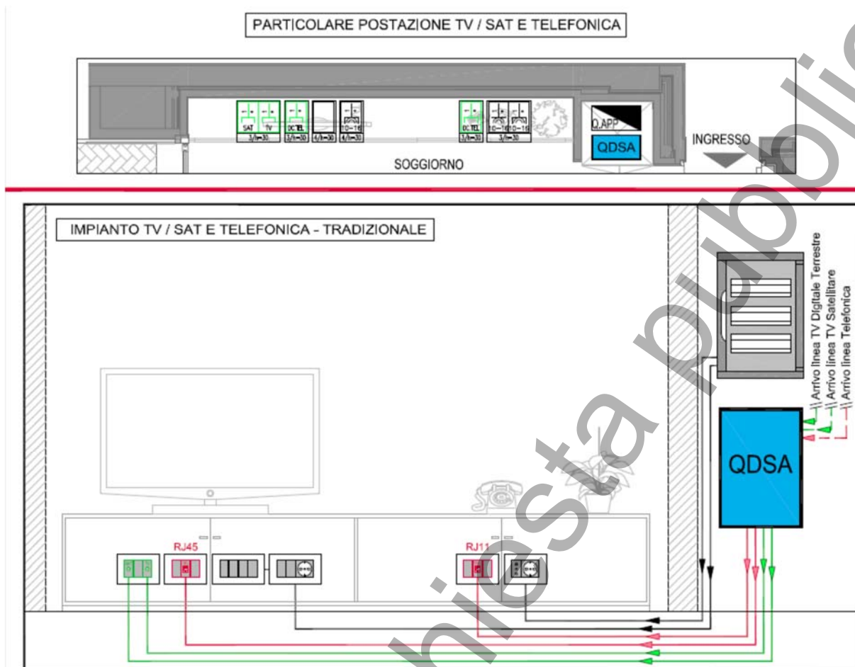
Figura 86 – Soggiorno: dettaglio postazione TV/SAT e fonia/dati
