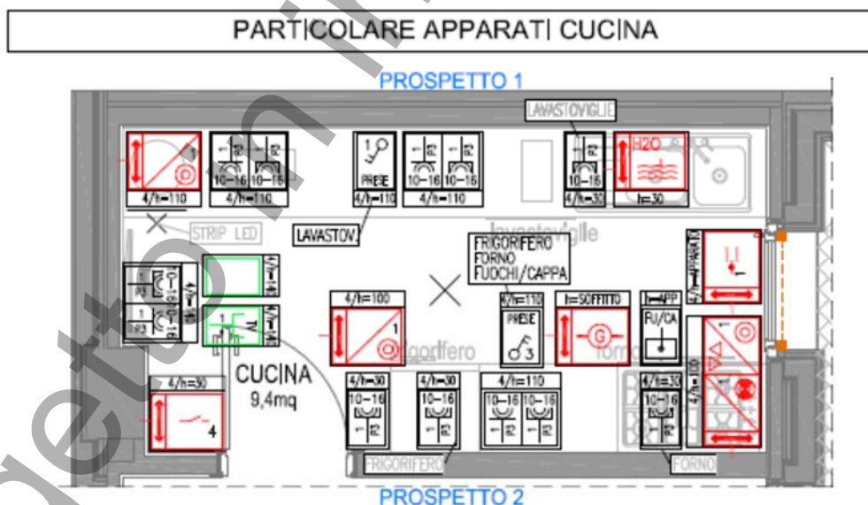
Figura 83 – Dettaglio cucina
