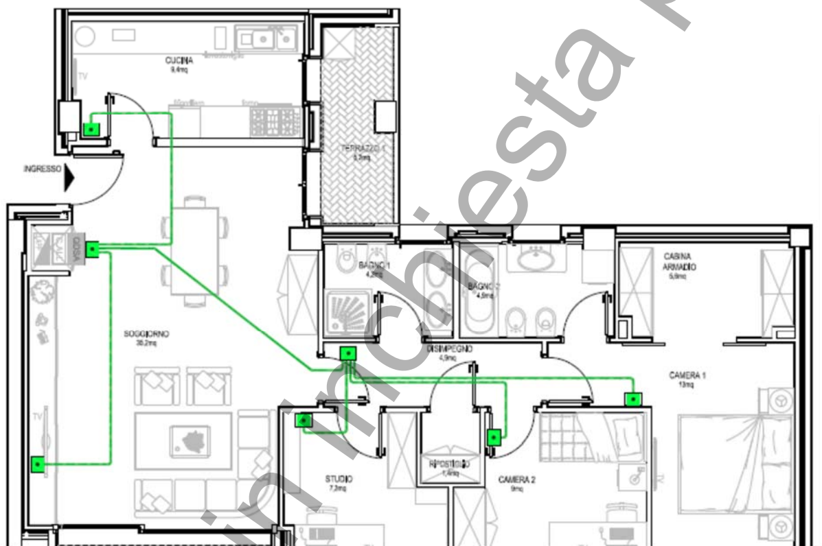
Figura 38 – Esempio di infrastruttura per impianti TV, fonia, trasmissione dati
